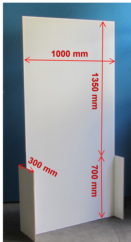
Ansicht Stellwand
